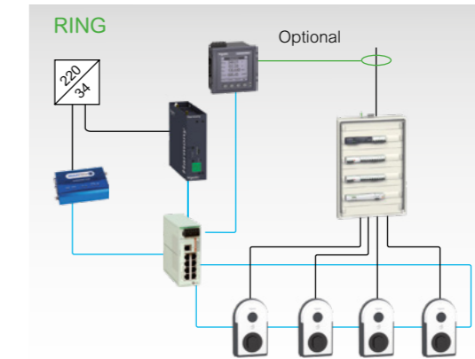
Ringschaltung mit einstellbarem Switch
