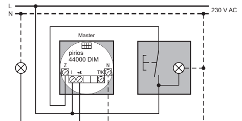
fig. 3 Fonction de poussoir Redéclenchement
