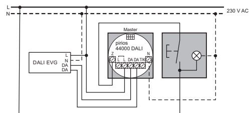
fig. 3 Fonction de poussoir Redéclenchement
