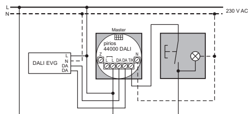
fig. 1 Fonction de poussoir Encl./Eco-Décl.
