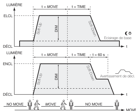
fig. 2 Eclairage de base / Préavertissement de coupure
