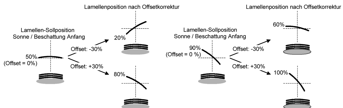
Bild 25: Funktionsweise des Lamellenoffsets als Beispiel (beispielhaft für Lamellentyp 1 / Lamellentyp 2 sinngemäß gleich)
