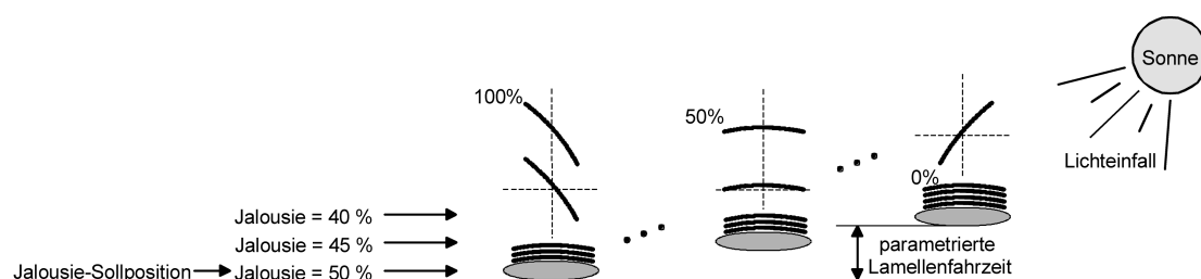
Bild 16: Beispiel für Lamellenpositionierung mit Auswirkung auf die Jalousieposition (Beispielhaft für Lamellentyp 1. Typ 2 sinngemäß gleich.)
