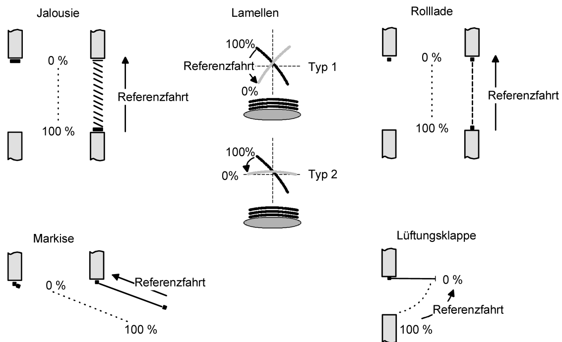
Bild 18: Referenzfahrt
