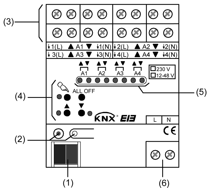
Bild 2: Geräteaufbau des Jalousieaktors 2/4fach REG
