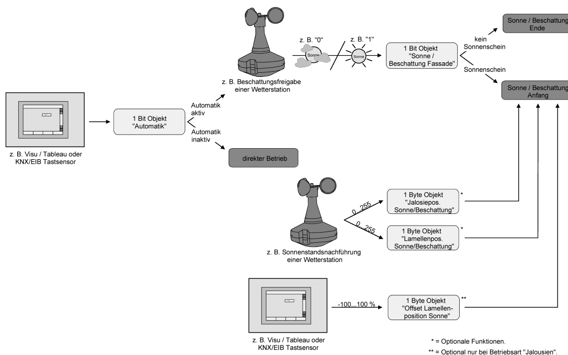
Bild 23: Prinzipschaltbild des erweiterten Sonnenschutzes (zur Vereinfachung ohne Sperrfunktionen)
