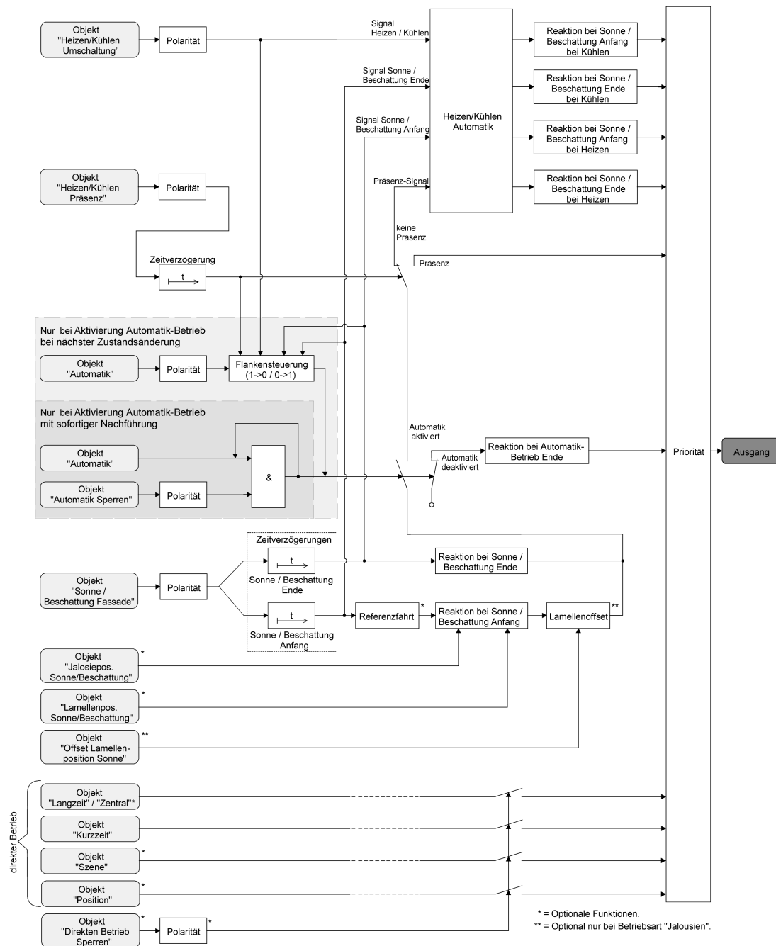
Bild 27: Funktionsschaltbild der Heizen/Kühlen-Automatik
