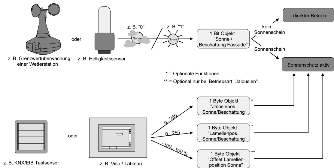
Bild 21: Prinzipschaltbild des einfachen Sonnenschutzes
