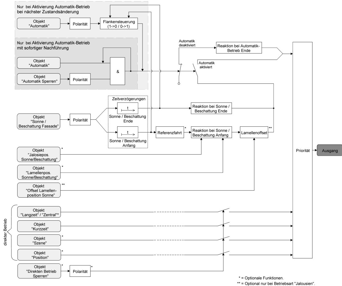
Bild 24: Funktionsschaltbild des erweiterten Sonnenschutzes
