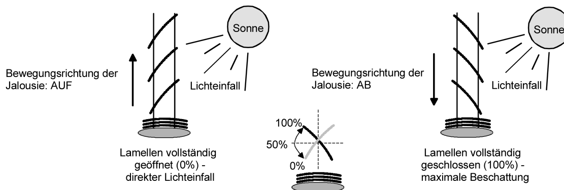
Bild 13: Typ 1 - Lamellenjalousien mit schräger Lamellenstellung in beide Fahrtrichtungen
