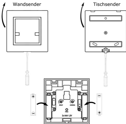
Fig. 1 Batterien einsetzen, auswechseln
