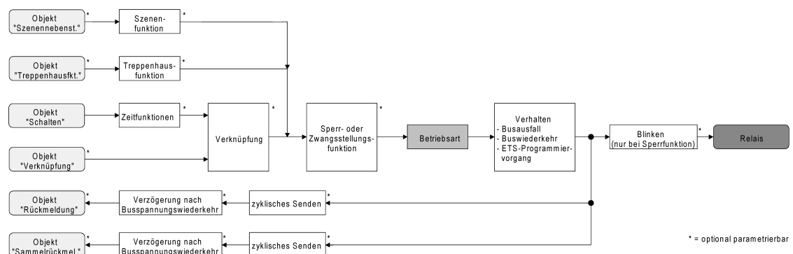
Bild 14: Funktionsschaltbild "Betriebsart"
