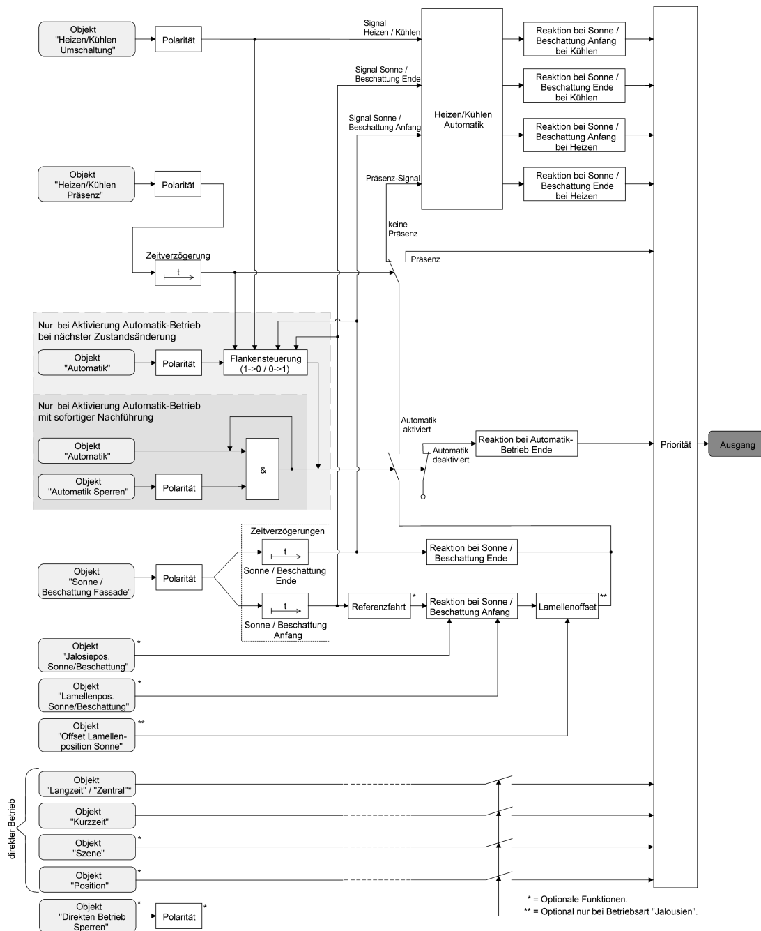
Bild 44: Funktionsschaltbild der Heizen/Kühlen-Automatik
