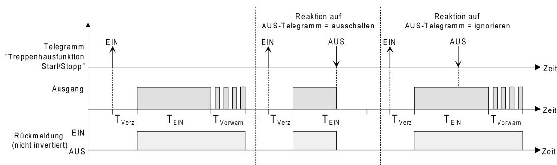
Bild 19: Ausschaltverhalten der Treppenhausfunktion
