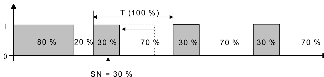
Bild 54: Stellgrößenänderung z. B. von 80 % auf 30 % während Öffnungsphase des Ventils
