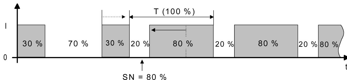
Bild 58: Stellgrößenänderung z. B. von 30 % auf 80 % während Schließphase des Ventils
