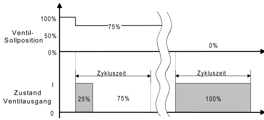
Bild 49: Umsetzung einer stetigen Ventil-Sollposition in ein Ausgangssignal bei stromlos geöffneten Ventilantrieben (Beispiel)
