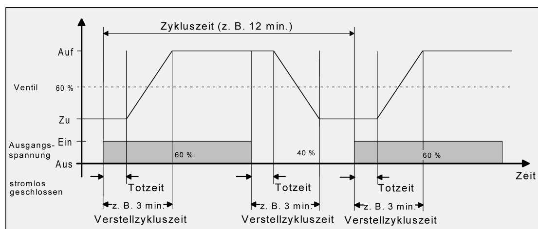
Bild 60: Idealisierter Verlauf des Ventilhubes exemplarisch dargestellt für eine Stellgröße von ca. 60 % eines stromlos geschlossenen Ventils
