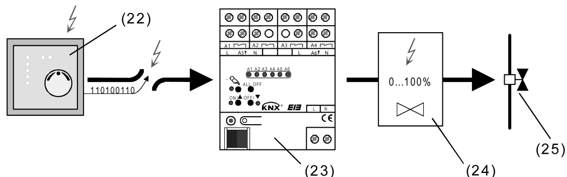
Bild 62: Prinzip der zyklischen Stellgrößenüberwachung im Störfall (z. B. Leitungsbruch)
