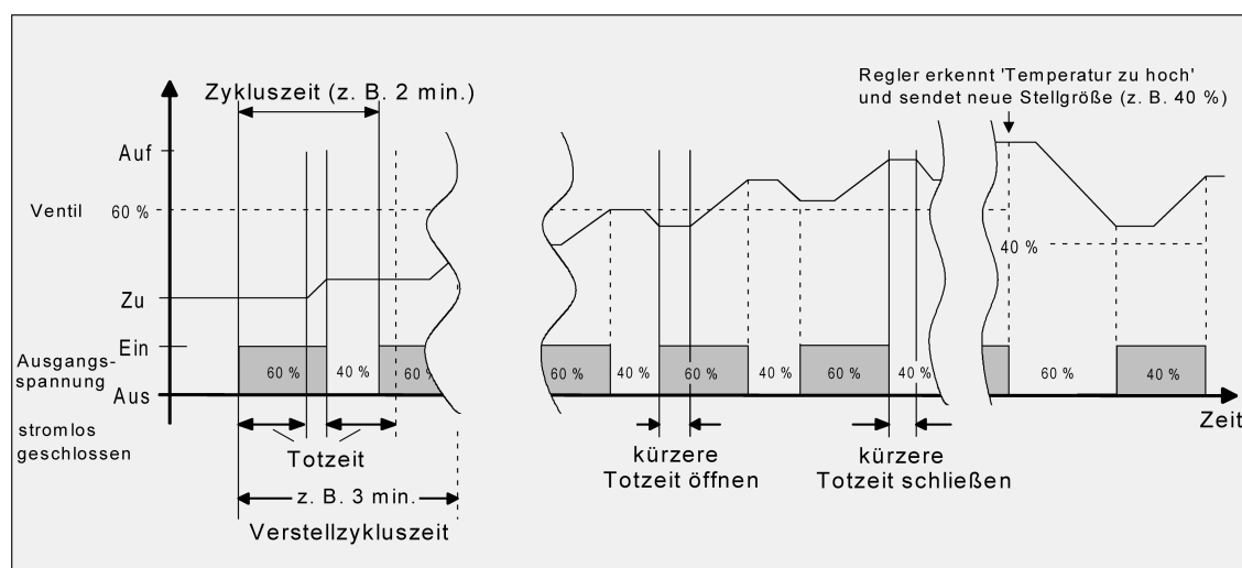
Bild 61: Idealisierter Verlauf des Ventilhubes exemplarisch dargestellt für eine Stellgröße von zunächst ca. 60 % eines stromlos geschlossenen Ventils
