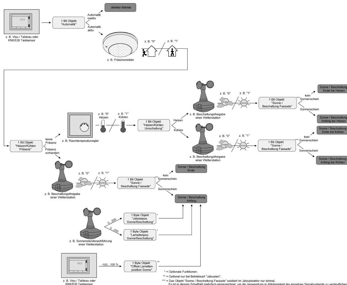
Bild 43: Prinzipschaltbild der Heizen/Kühlen-Automatik (zur Vereinfachung ohne Sperrfunktionen des Automatik-Betriebs oder des direkten Betriebs)
