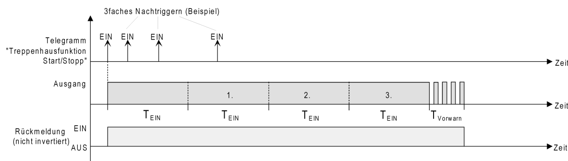
Bild 21: Zeitverlängerung der Treppenhausfunktion
