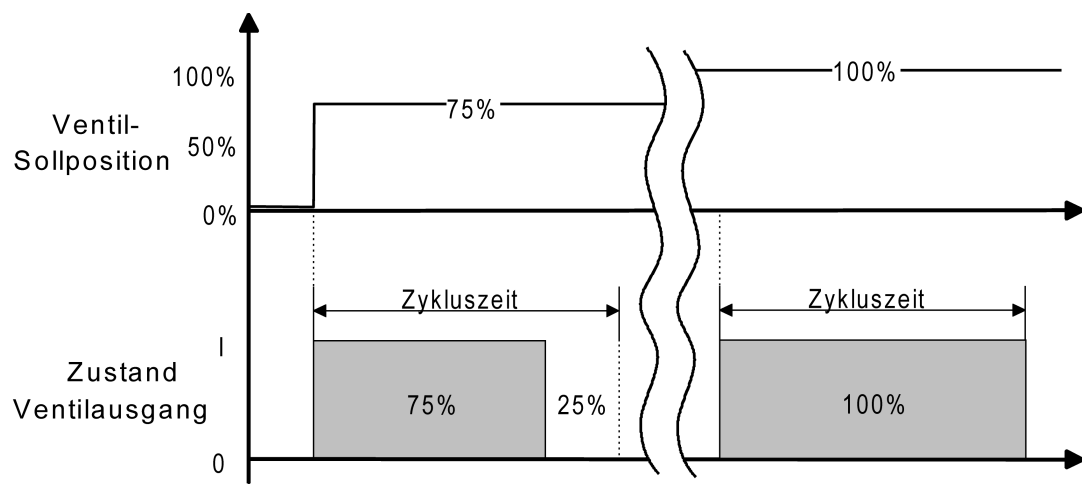
Bild 47: Umsetzung einer stetigen Ventil-Sollposition in ein Ausgangssignal bei stromlos geschlossenen Ventilantrieben (Beispiel)
