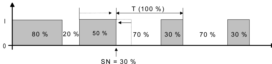
Bild 56: Stellgrößenänderung z. B. von 80 % auf 30 % während Öffnungsphase des Ventils (Öffnungsphase zu lang)
