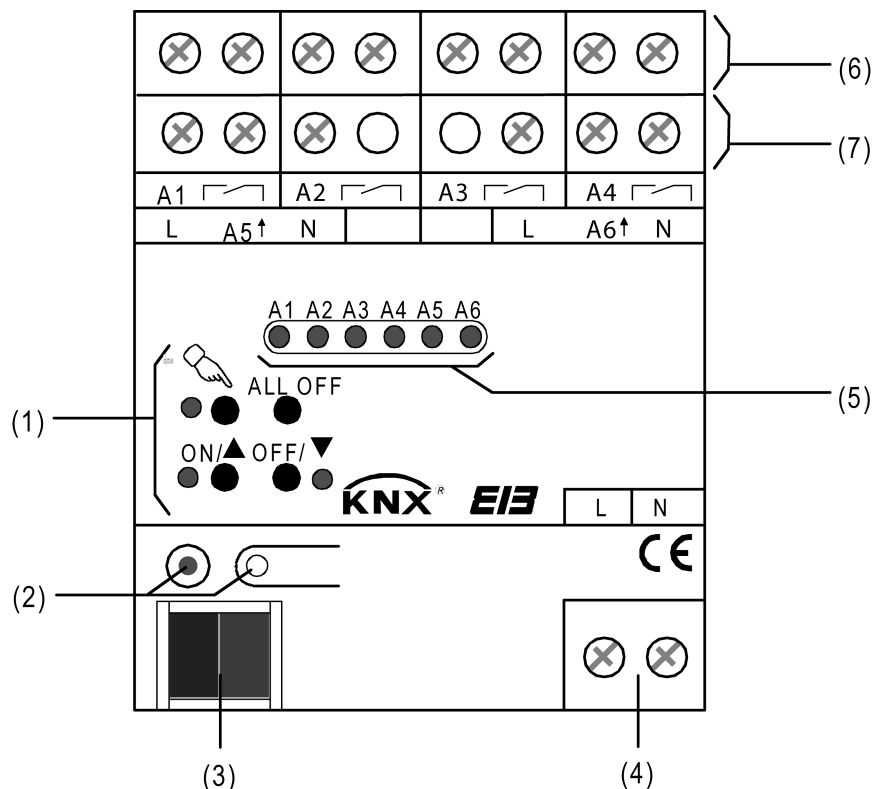
Bild 1: Geräteaufbau
