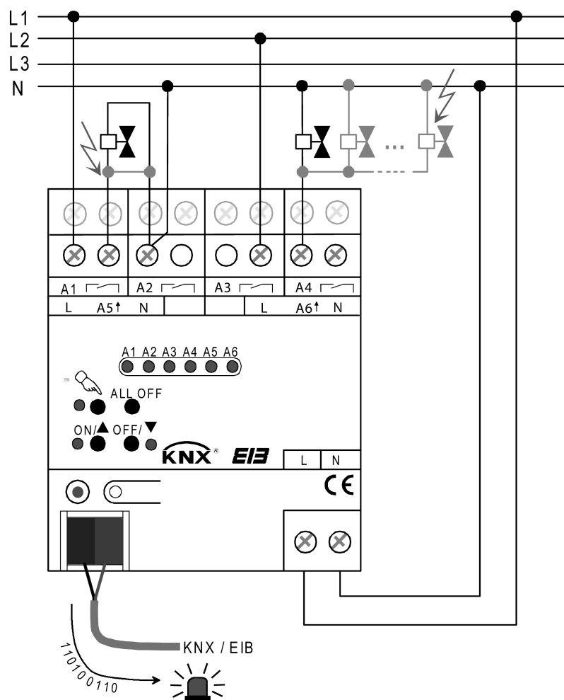
Bild 50: Kurzschluss- und Überlasterkennung bei Störung eines Ventilausgangs oder Ventiltriebs
