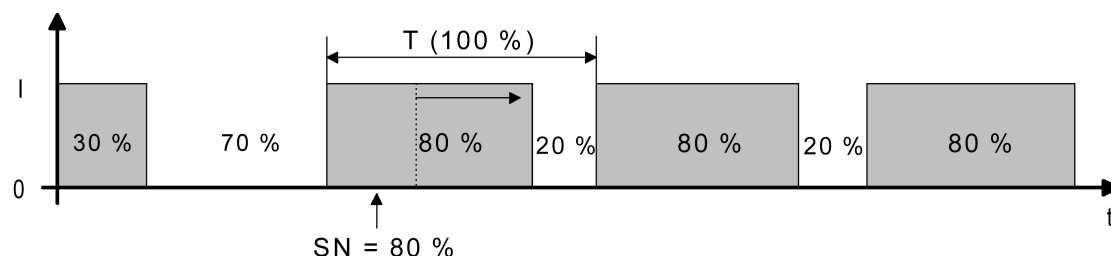
Bild 57: Stellgrößenänderung z. B. von 30 % auf 80 % während Öffnungsphase des Ventils
