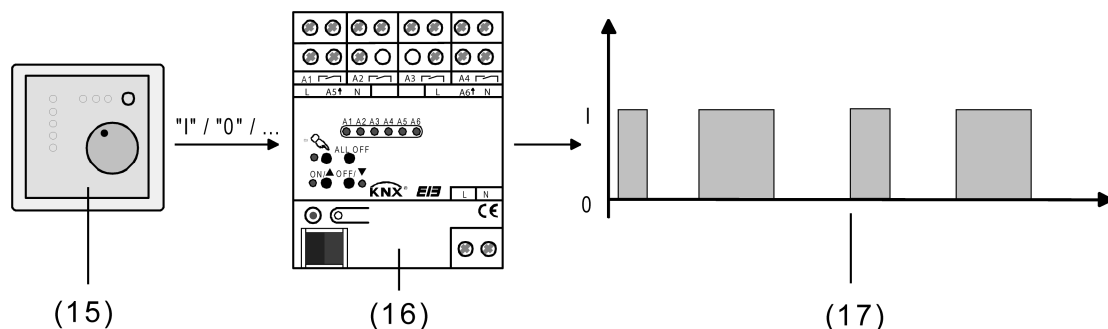
Bild 51: Stellgrößenprinzip bei schaltender Stellgröße
