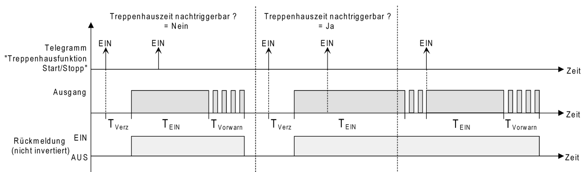
Bild 18: Einschaltverhalten der Treppenhausfunktion
