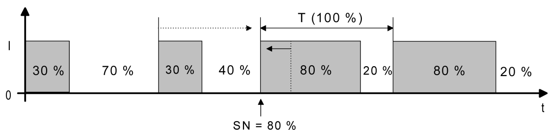
Bild 59: Stellgrößenänderung z. B. von 30 % auf 80 % während Schließphase des Ventils (Schließphase zu lang)
