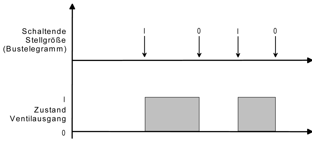
Bild 46: Umsetzung einer schaltenden Stellgröße in ein Ausgangssignal bei stromlos geschlossenen Ventilantrieben (Beispiel)
