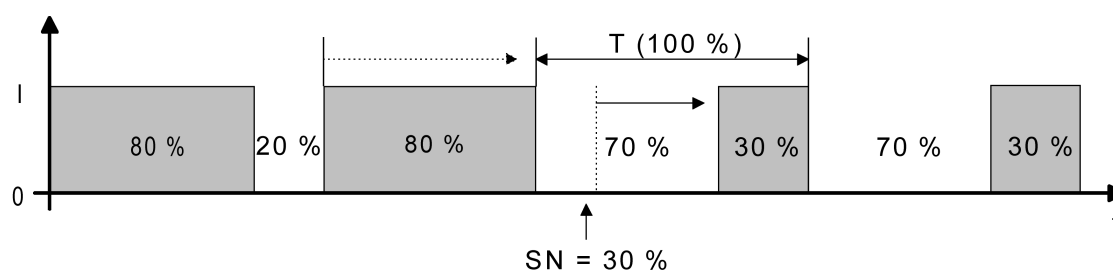
Bild 55: Stellgrößenänderung z. B. von 80 % auf 30 % während Schließphase des Ventils
