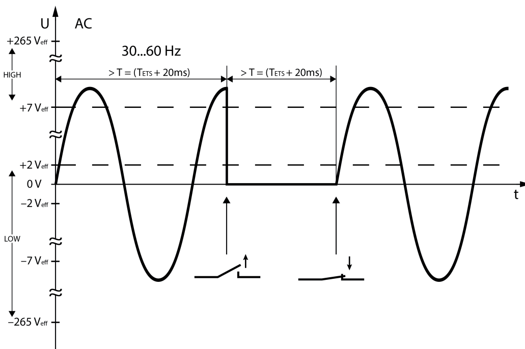
Bild 7: Beispiel eines Signalverlaufes eines Wechselspannungssignals (AC)
