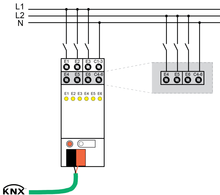
Bild 2: Anschluss netzversorgter Stromkreise
