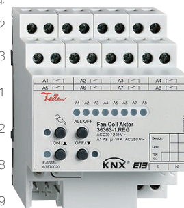
Attuatore FanCoil Feller 36363-1.REG
