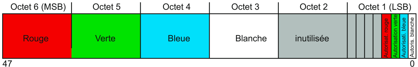
Figure 31: Type de données KNX "RGBW combiné" (DPT 251.600)
