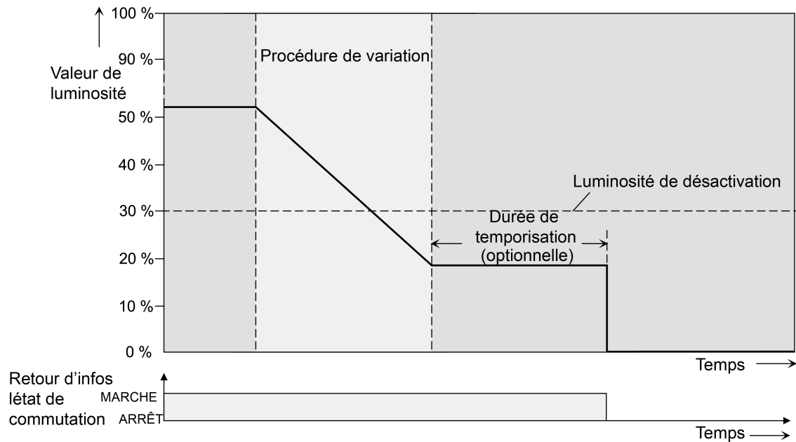
Figure 46: Comportement de variation et de commutation de la fonction de désactivation automatique
