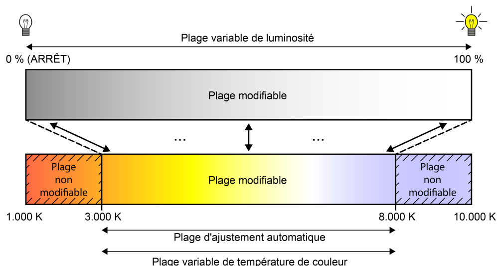
Figure 25: Adaptation automatique de la température de couleur à la luminosité réglée
