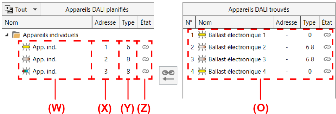
Figure 70: Exemple d'appareils individuels DALI configurés dans la zone d'affichage de gauche
