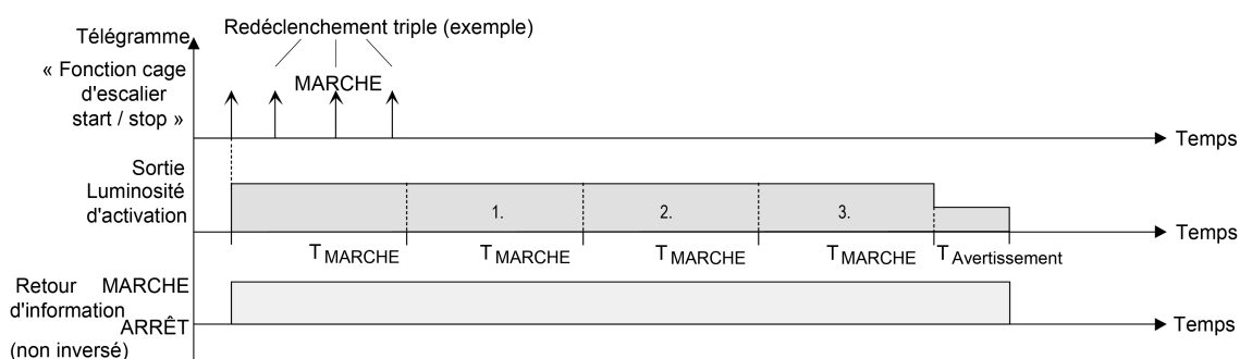
Figure 55: Prolongation de la fonction cage d'escalier
