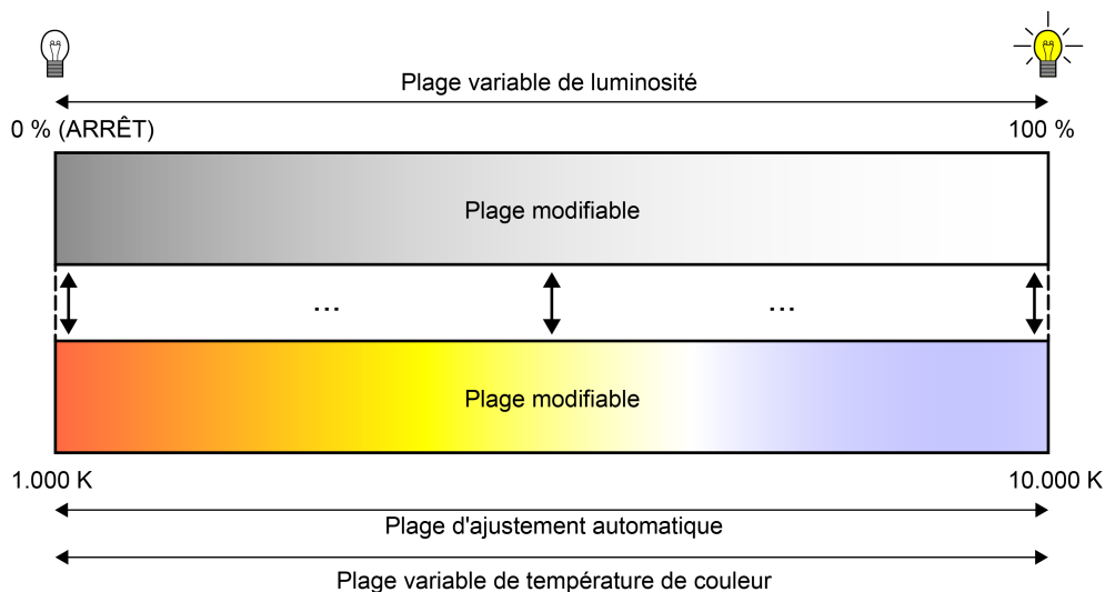
Figure 23: Adaptation automatique de la température de couleur à la luminosité réglée Exemple dans la plage de luminosité et de température de couleur maximale
