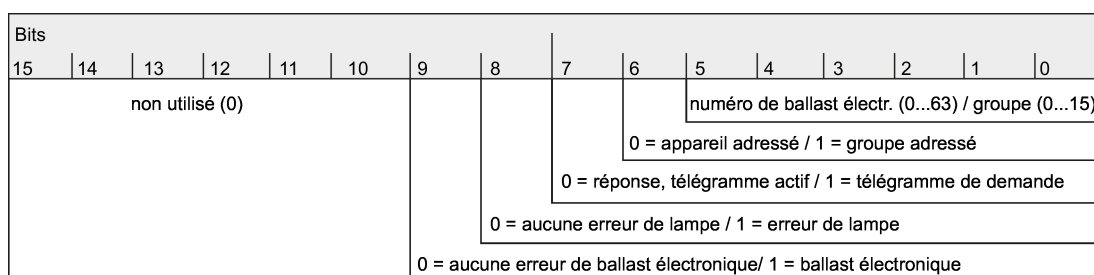
Figure 13: Structure du télégramme État d'erreur 2 octet
