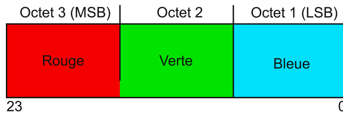
Figure 30: Type de données KNX "RGB combiné" (DPT 232.600)
