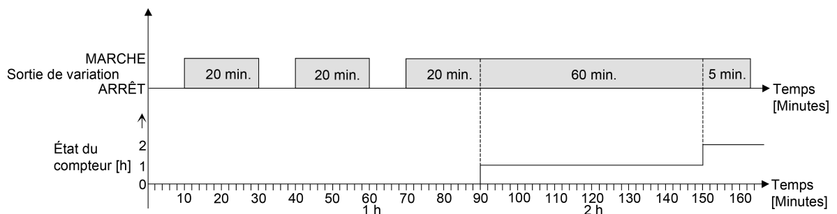
Figure 56: Mode de fonctionnement du compteur d'heures de fonctionnement (sur l'exemple : heures comptées)
