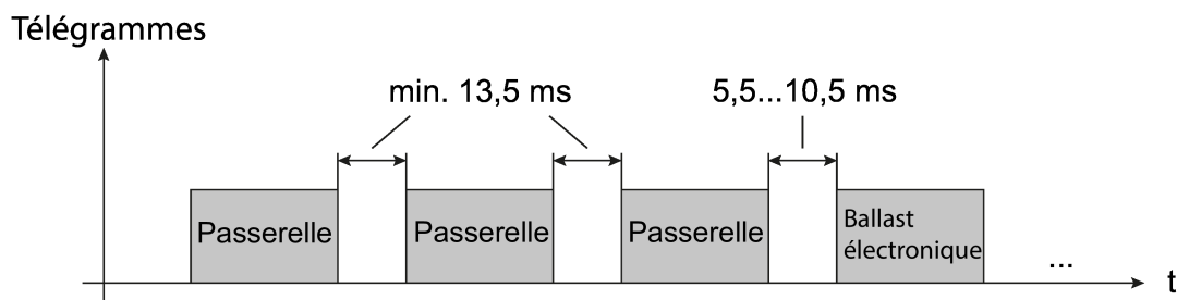
Figure 10: Temps de pause entre les instructions DALI
