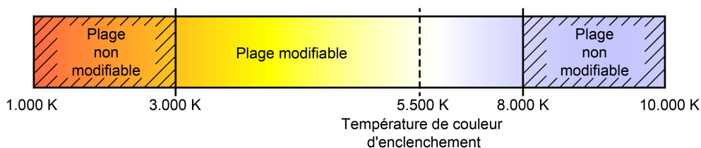
Figure 21: Exemple d'une plage de température de couleur configurée avec une température de couleur d'enclenchement
