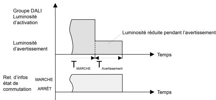
Figure 51: La fonction d'avertissement de la fonction cage d'escalier sans fonction ARRÊT progressif
