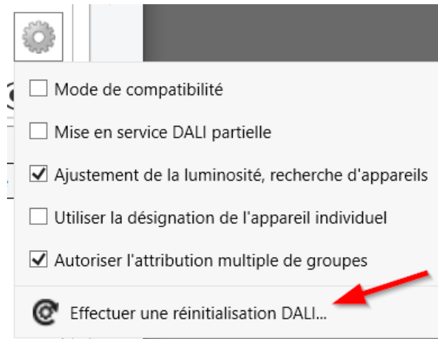
Figure 73: Instruction de réinitialisation DALI dans le menu contextuel de la mise en service DALI
