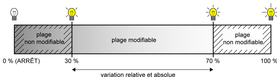
Figure 16: Exemple d'une plage de luminosité à intensité variable
