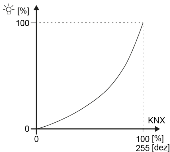
Figure 20: Courbe de variation combinée à la sortie d'un équipement (flux lumineux relatif [%] en fonction de la valeur de données KNX de 8 bits [0...255])
