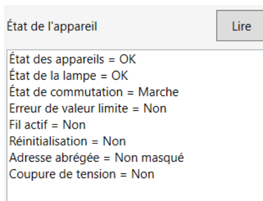
Figure 78: Exemple d'état de l'appareil
