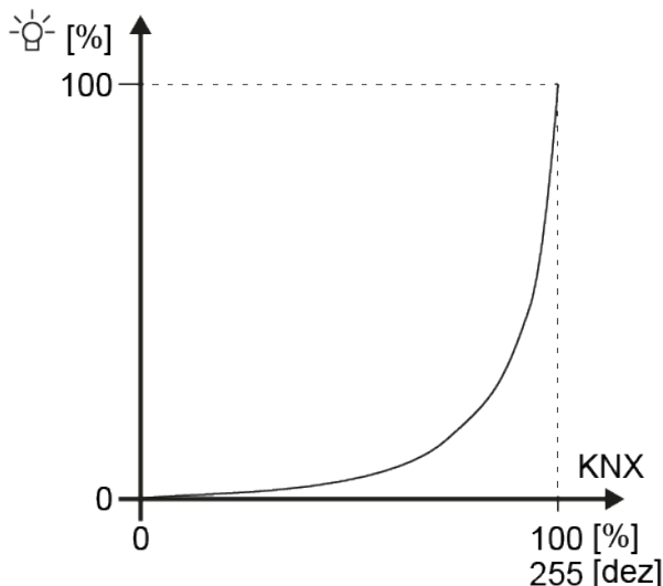
Figure 19: Courbe de variation logarithmique à la sortie d'un équipement (flux lumineux relatif [%] en fonction de la valeur de données KNX de 8 bits [0...255])
