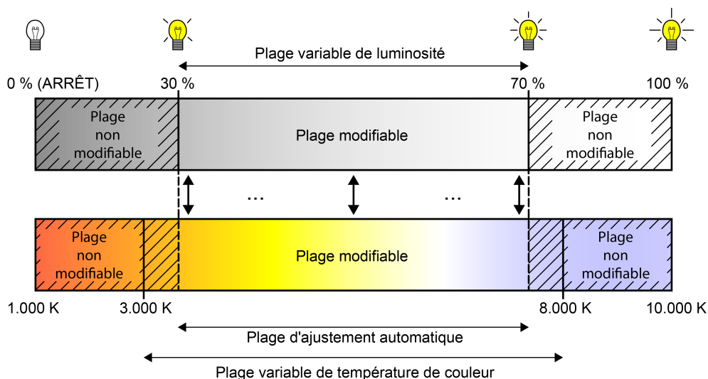
Figure 24: Adaptation automatique de la température de couleur à la luminosité réglée Exemple avec une plage de luminosité et de température de couleur restreinte
