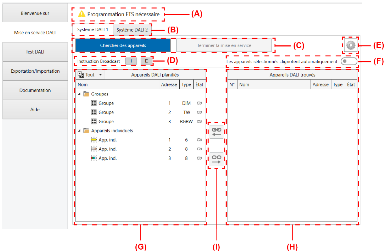
Figure 59: Environnement de mise en service DALI dans la DCA
