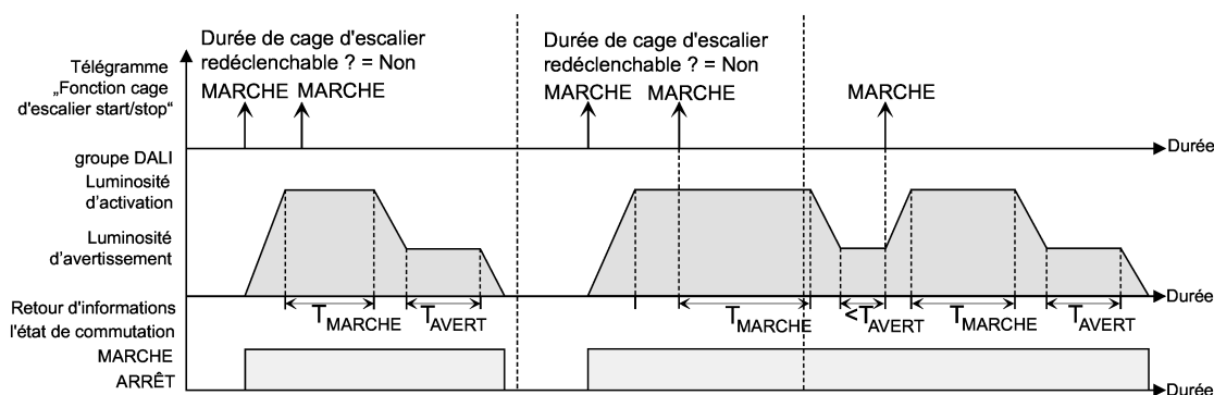
Figure 48: Comportement d'activation de la fonction cage d'escalier avec fonctions progressives (exemple avec luminosité minimale = 0 %)
