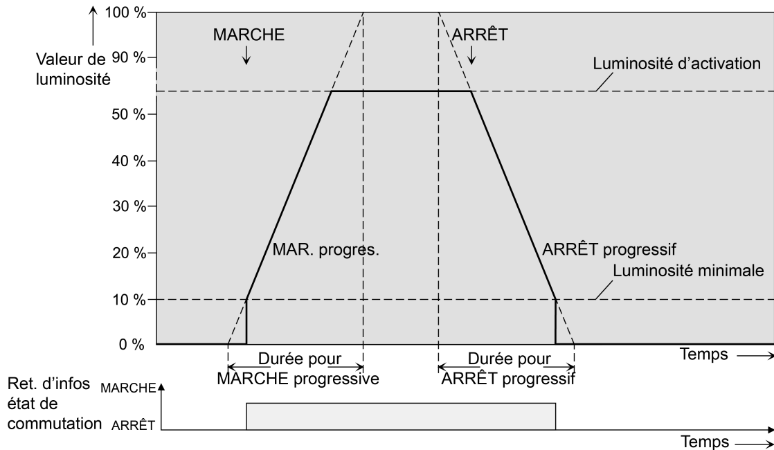
Figure 45: Exemple de comportement de variation des fonctions MARCHÉ progressive / ARRÊT progressif avec luminosité minimale > 0 %
