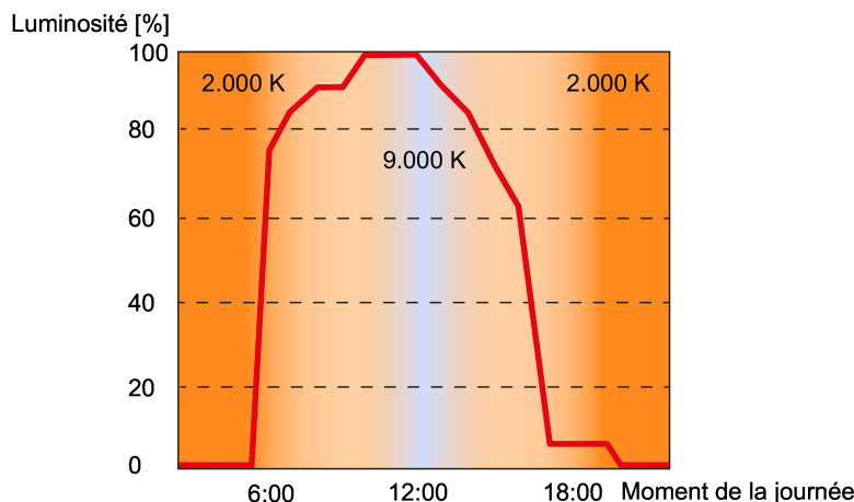
Figure 28: Exemple de dégradé de température de couleur du jour "Santé et soins"
