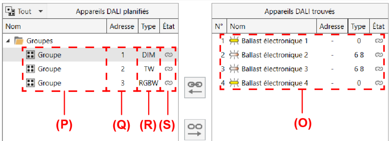
Figure 66: Exemple de groupes DALI configurés dans la zone d'affichage de gauche
