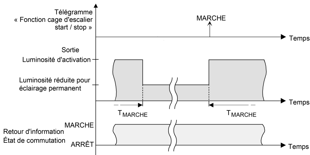
Figure 53: Éclairage permanent de la fonction cage d'escalier sans fonctions progressives
