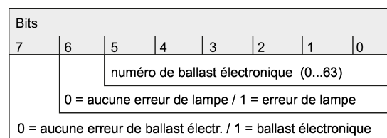
Figure 12: Structure du télégramme État d'erreur 1 octet
