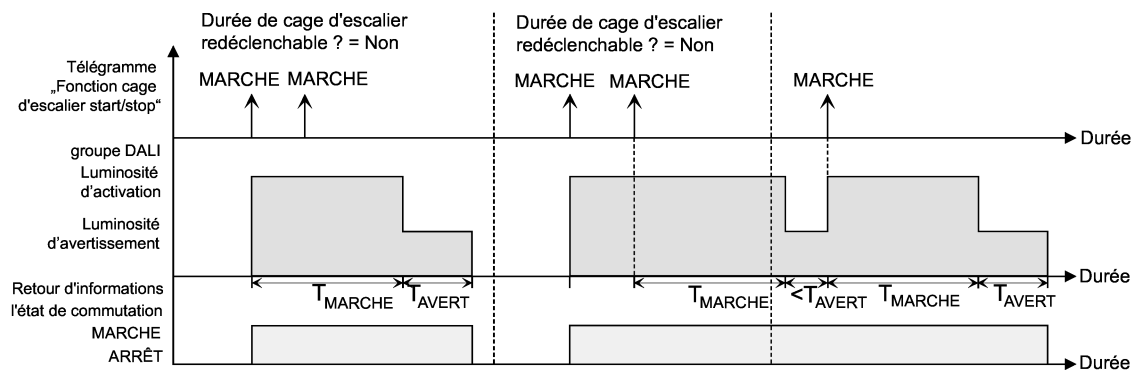
Figure 47: Comportement d'activation de la fonction cage d'escalier sans fonctions progressives
