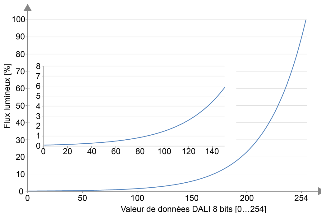
Figure 17: Courbe de variation logarithmique dans des équipements DALI (flux lumineux relatif [%] en fonction de la valeur de données DALI de 8 bits [0...254])
