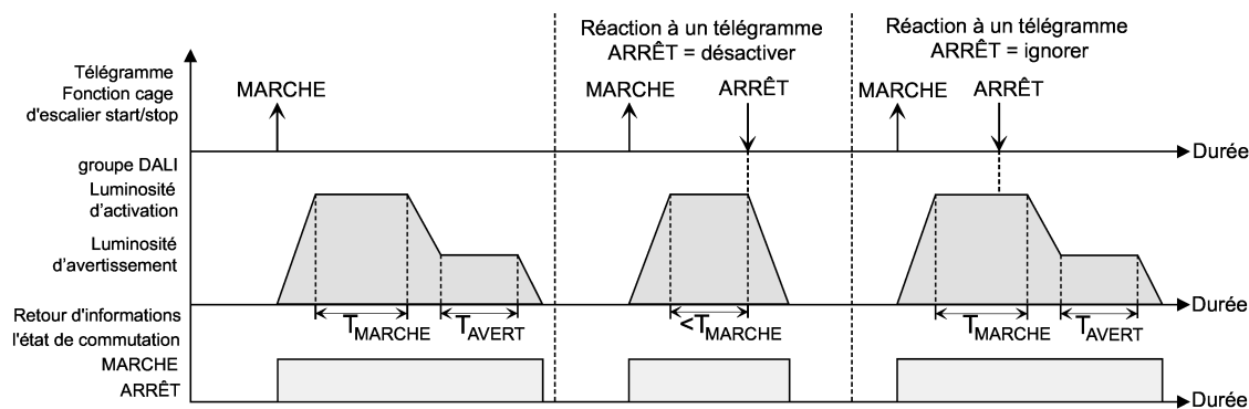
Figure 50: Comportement de désactivation de la fonction cage d'escalier avec fonctions progressives (exemple avec luminosité minimale = 0 %)
