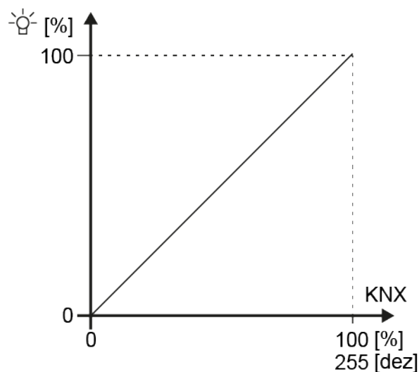
Figure 18: Courbe linéaire de variation à la sortie d'un dispositif (flux lumineux relatif [%] en fonction de la valeur de données KNX de 8 bits [0...255])
